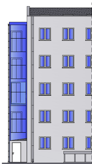
ELEWACJA BOCZNA
